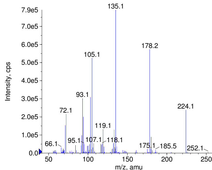
+ Meperidine-D4 Prec(252.0) CE(50.0) RT(0.9)
