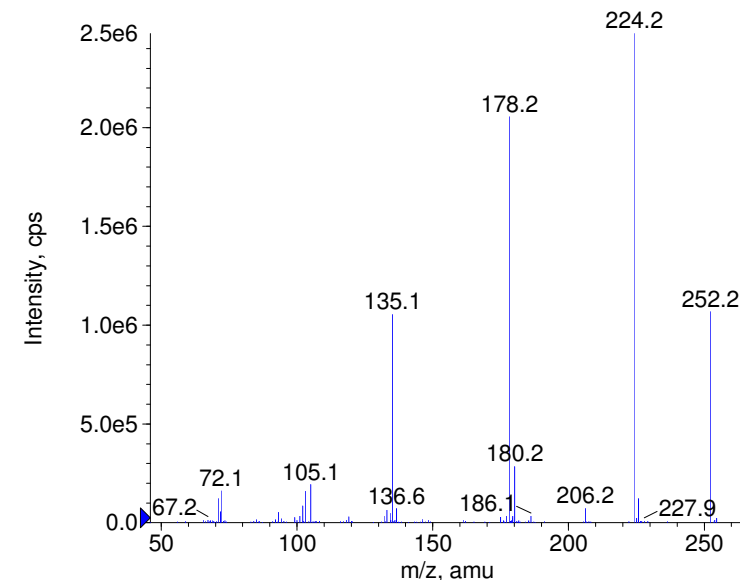
+ Meperidine-D4 Prec(252.0) CE(99.0) RT(0.9)
