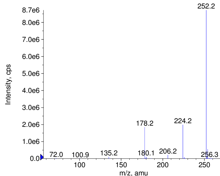
+ Meperidine-D4 Prec(252.0) CE(50.0) RT(0.9)
