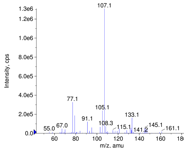
+ Meptazinol Prec(234.0) CE(50.0) RT(0.8)
