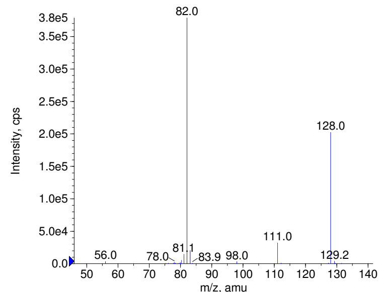
+ Metronidazole Prec(172.0) CE(99.0) RT(0.7)
