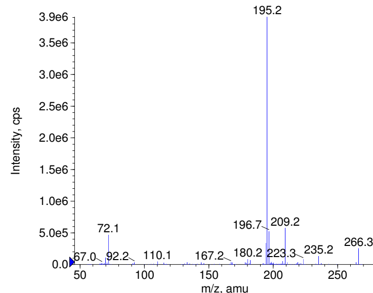
+ Mirtazapine Prec(266.0) CE(99.0) RT(0.7)
