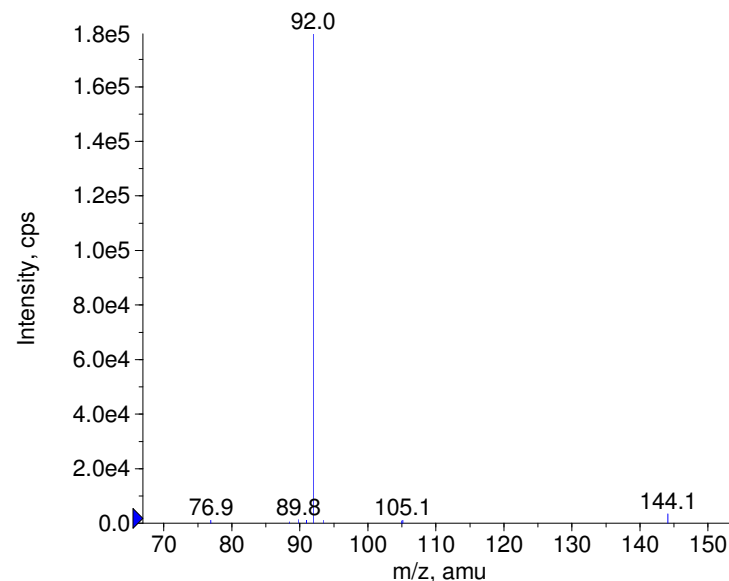
■ - Mofebutazone Prec(231.0) CE(-50.0) RT(0.9)
