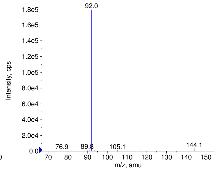
■ - Mofebutazone Prec(231.0) CE(-50.0) RT(0.9)
