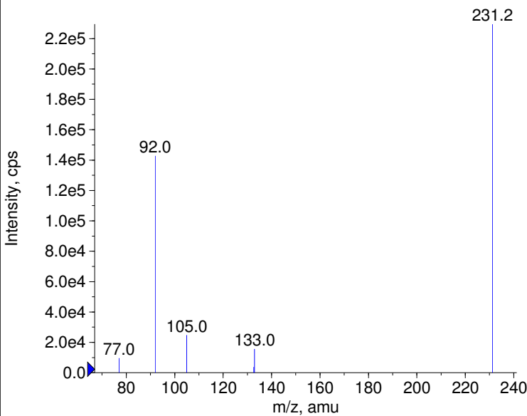
■ - Mofebutazone Prec(231.0) CE(-99.0) RT(1.0)
