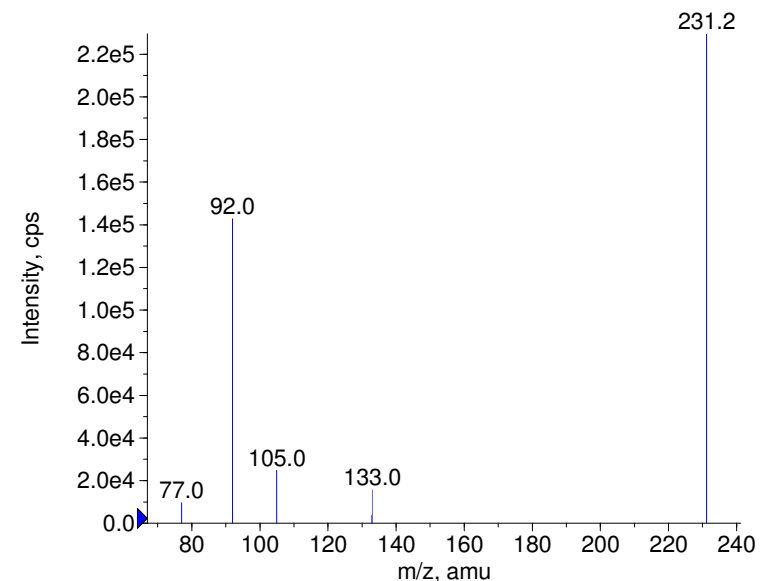
■ - Mofebutazone Prec(231.0) CE(-99.0) RT(1.0)
