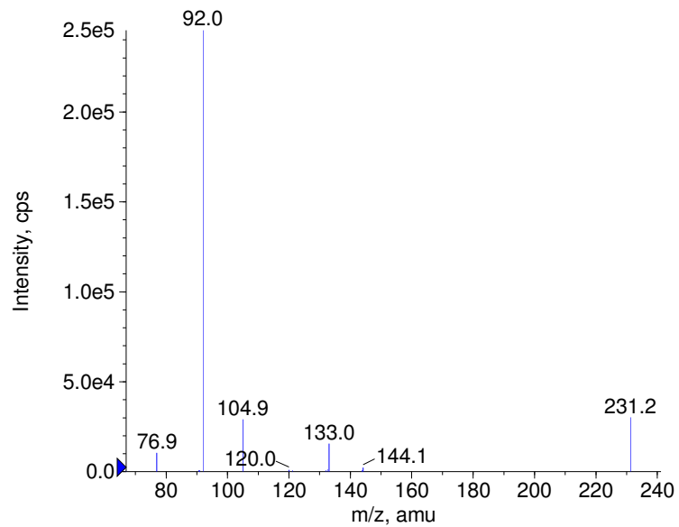
■ - Mofebutazone Prec(231.0) CE(-35.0) RT(0.9)
