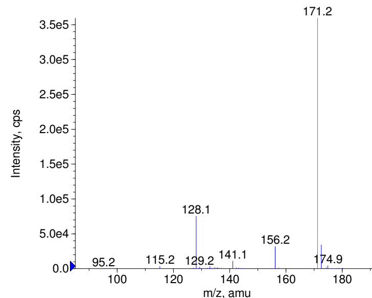
+ Nabumetone Prec(229.0) CE(99.0) RT(1.3)
