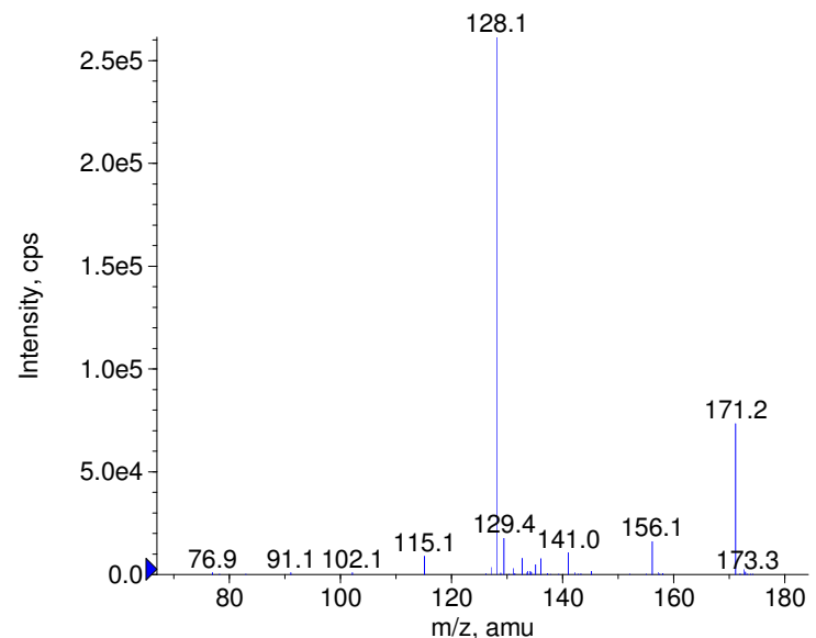
+ Nabumetone Prec(229.0) CE(50.0) RT(1.2)
