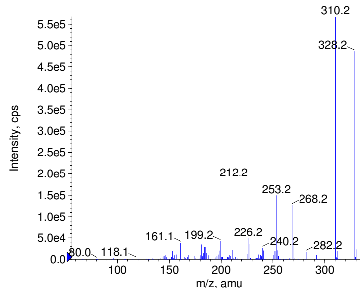
+ Naloxone Prec(328.0) CE(99.0) RT(0.7)
