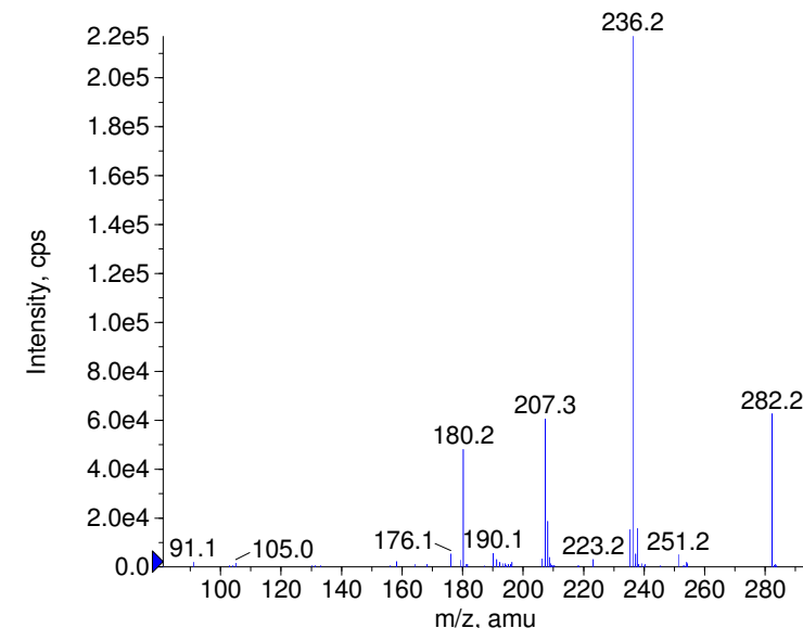
+ Nitrazepam Prec(282.0) CE(99.0) RT(0.9)
