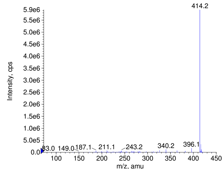
+ Norbuprenorphine Prec(414.0) CE(99.0) RT(0.8)
