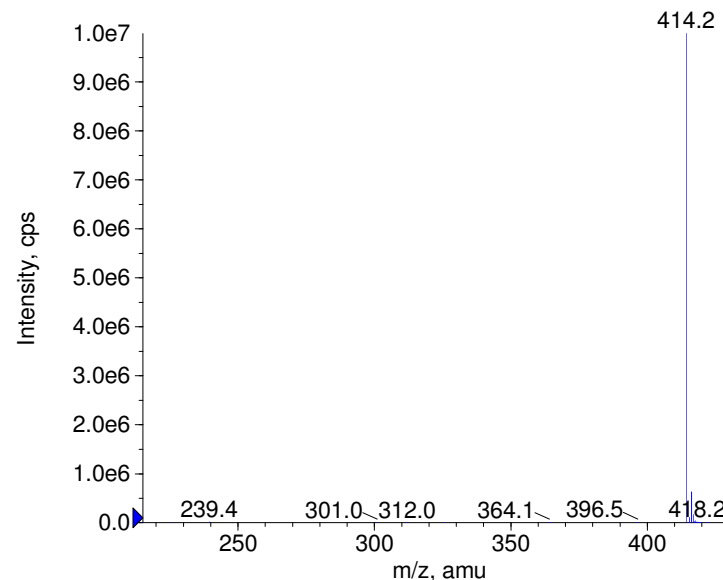
+ Norbuprenorphine Prec(414.0) CE(50.0) RT(0.8)
