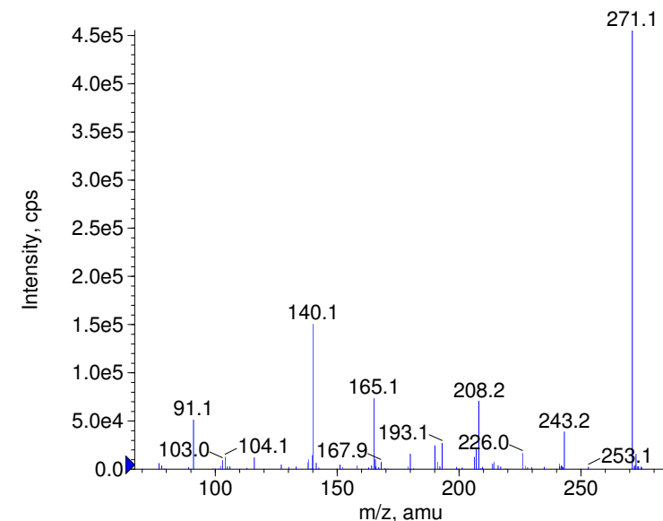
+ Nordiazepam Prec(271.0) CE(99.0) RT(1.0)
