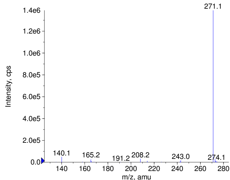
+ Nordiazepam Prec(271.0) CE(50.0) RT(1.0)
