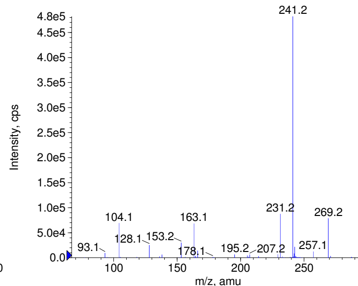
+ Oxazepam Prec(287.0) CE(99.0) RT(0.8)
