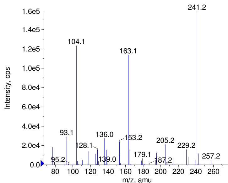
+ Oxazepam Prec(287.0) CE(50.0) RT(0.8)
