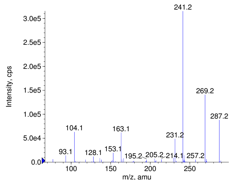
+ Oxazepam Prec(287.0) CE(99.0) RT(0.8)
