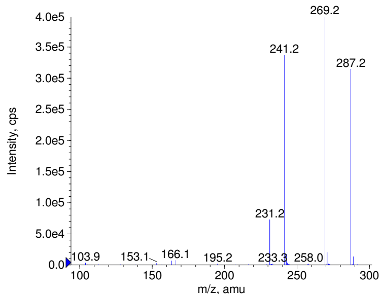
+ Oxazepam Prec(287.0) CE(50.0) RT(0.8)
