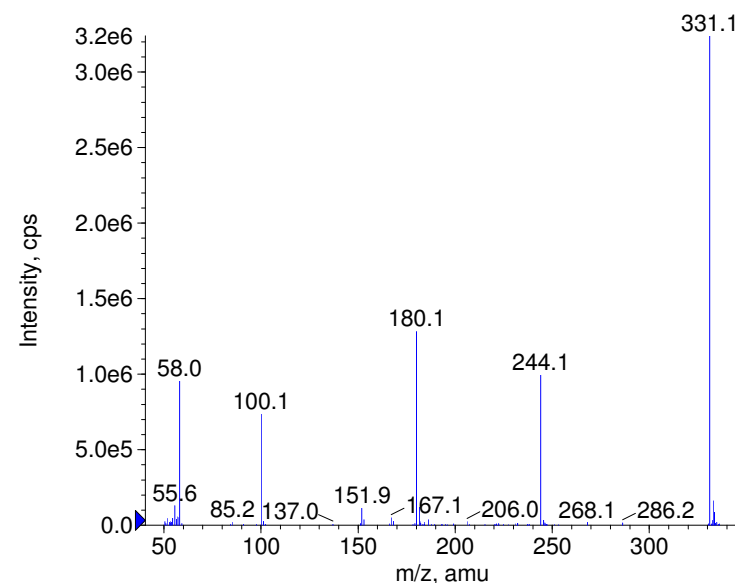
+ Oxomemazine Prec(331.0) CE(99.0) RT(0.8)
