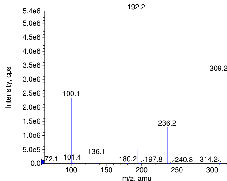
+ Oxybuprocaine Prec(309.0) CE(50.0) RT(0.8)
