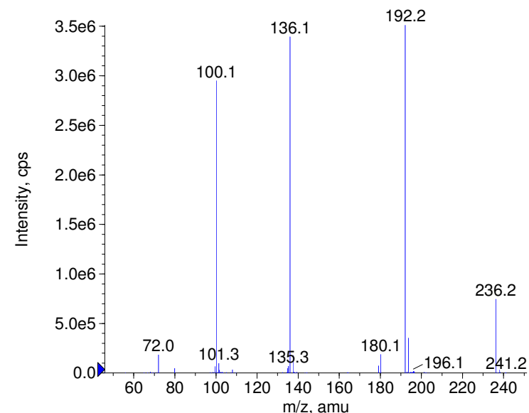
+ Oxybuprocaine Prec(309.0) CE(99.0) RT(0.8)
