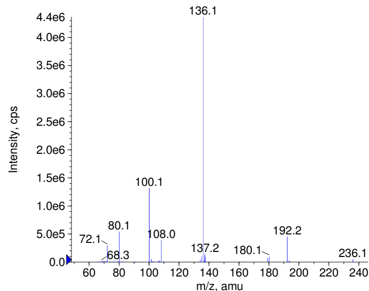
+ Oxybuprocaine Prec(309.0) CE(50.0) RT(0.8)
