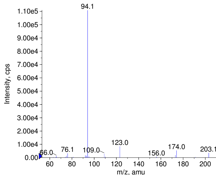
■ + Paraoxon Prec(276.0) CE(50.0) RT(0.9)
