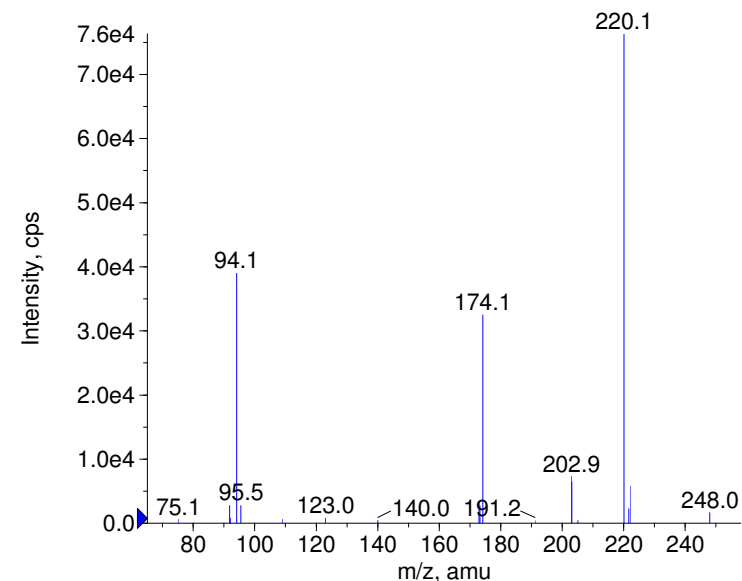
■ + Paraoxon Prec(276.0) CE(99.0) RT(1.0)
