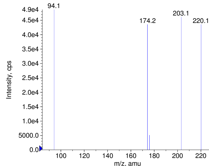
■ + Paraoxon Prec(276.0) CE(99.0) RT(1.0)
