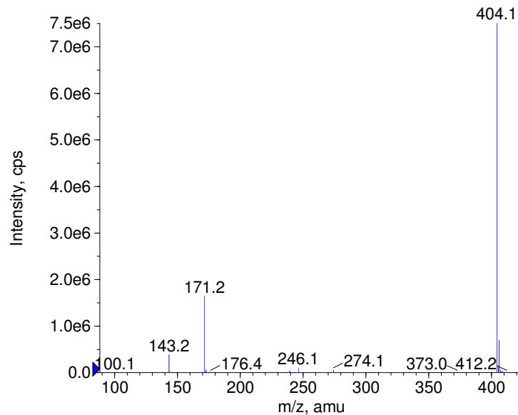
■ + Perphenazine Prec(404.0) CE(50.0) RT(0.7)
