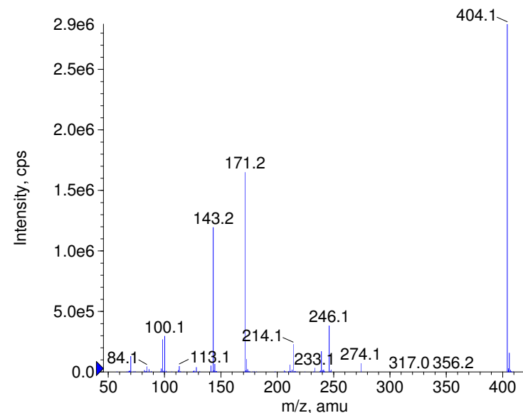
■ + Perphenazine Prec(404.0) CE(99.0) RT(0.7)
