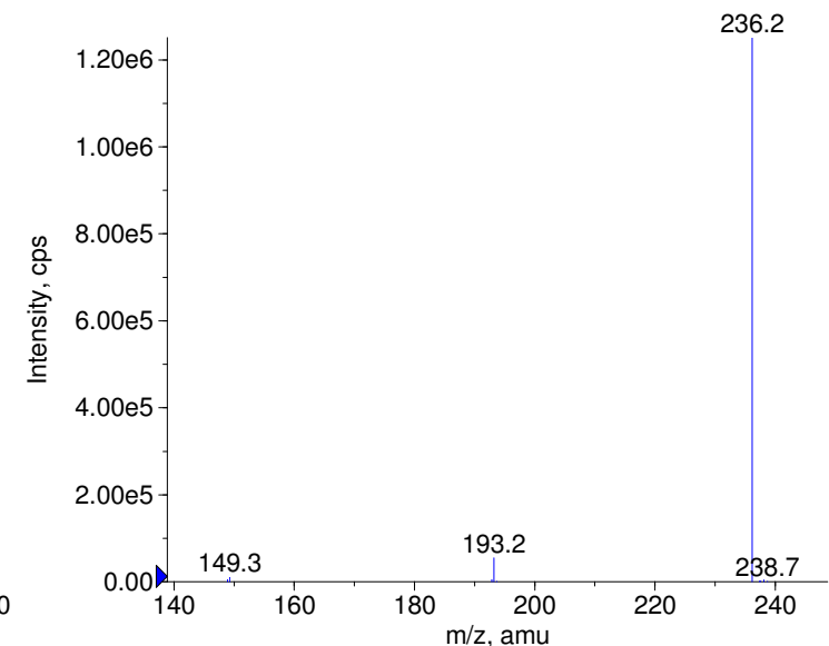
■ - Phenobarbital-D5 Prec(236.0) CE(-99.0) RT(0.9)
