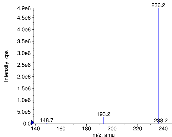
■ - Phenobarbital-D5 Prec(236.0) CE(-50.0) RT(0.9)
