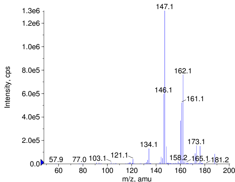
+ Physostigmine Prec(276.0) CE(50.0) RT(0.8)
