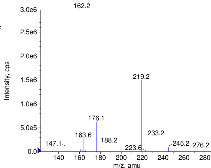
+ Physostigmine Prec(276.0) CE(50.0) RT(0.8)
