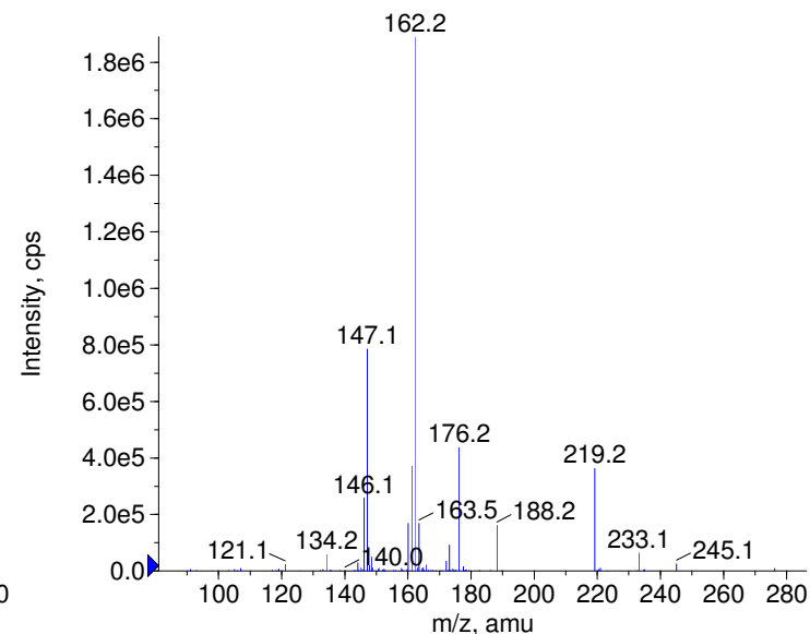
+ Physostigmine Prec(276.0) CE(99.0) RT(0.8)
