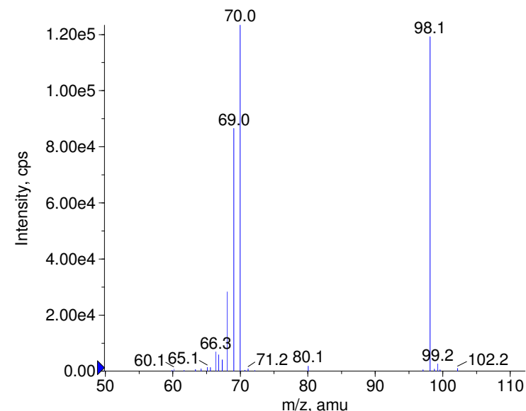
■ + Piracetam Prec(143.0) CE(99.0) RT(1.0)
