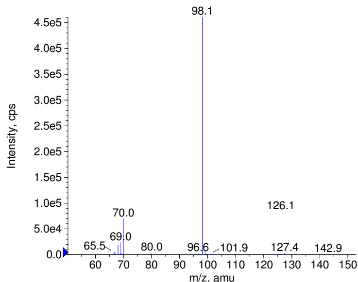
■ + Piracetam Prec(143.0) CE(50.0) RT(1.0)
