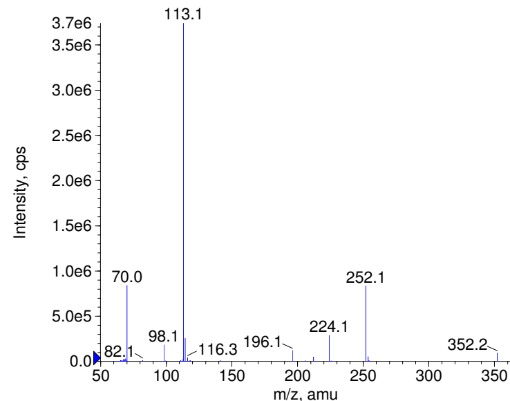
+ Pirenzepine Prec(352.0) CE(99.0) RT(0.8)
