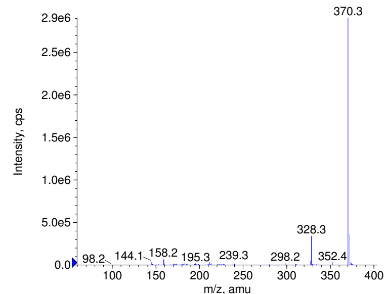
+ Prajmalium Prec(370.0) CE(99.0) RT(0.8)
