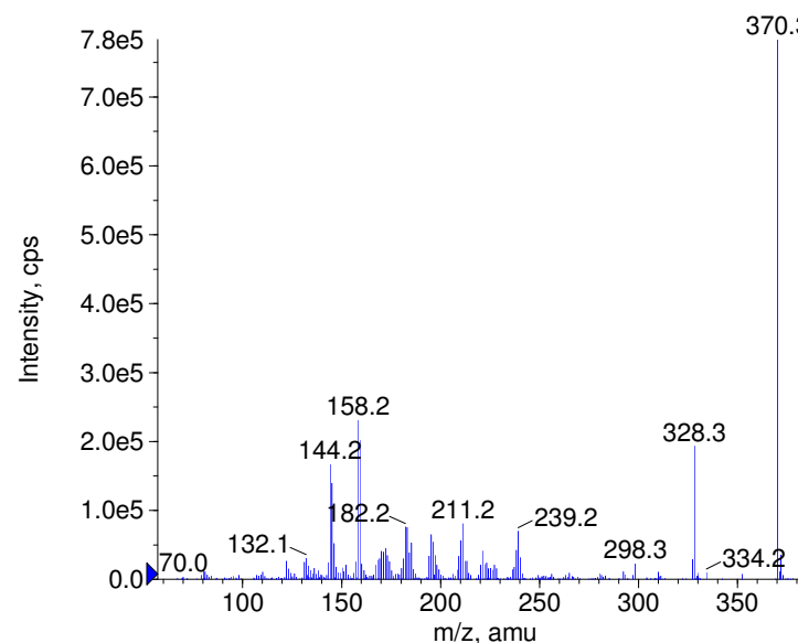
+ Prajmalium Prec(370.0) CE(50.0) RT(0.8)
