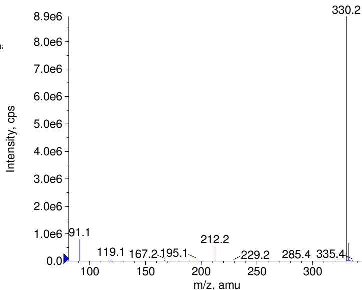
+ Prenylamine Prec(330.0) CE(50.0) RT(0.8)
