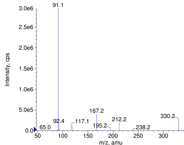
+ Prenylamine Prec(330.0) CE(99.0) RT(0.8)
