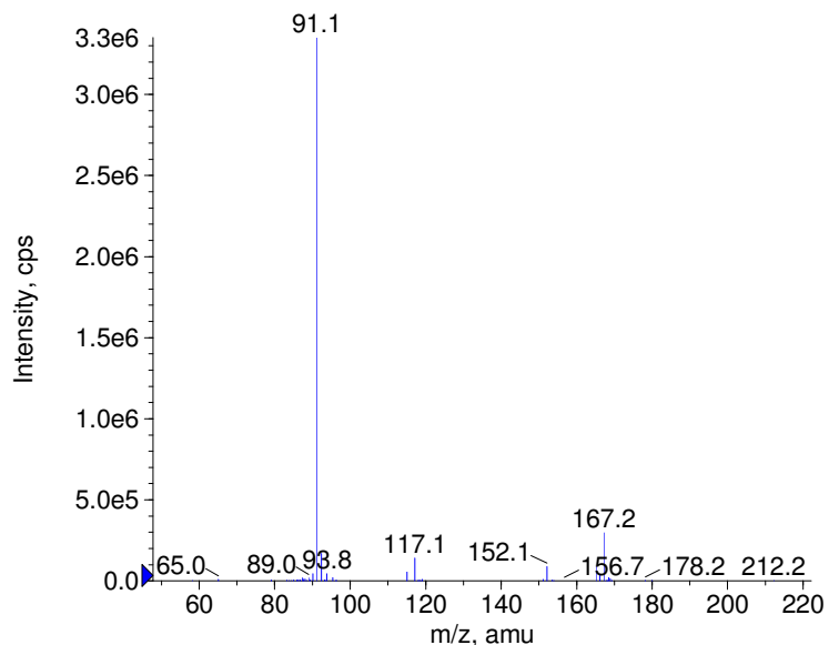
+ Prenylamine Prec(330.0) CE(50.0) RT(0.8)
