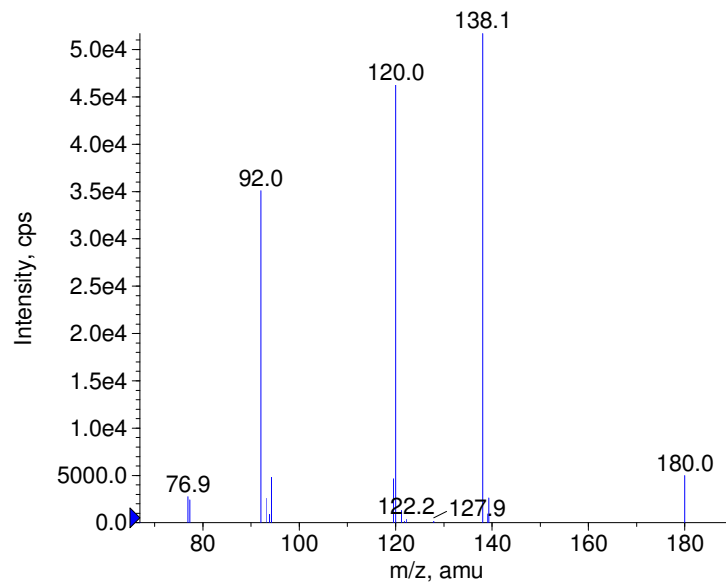
+ Propham Prec(180.0) CE(50.0) RT(0.6)
