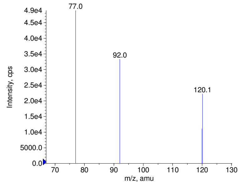
+ Propham Prec(180.0) CE(99.0) RT(0.6)
