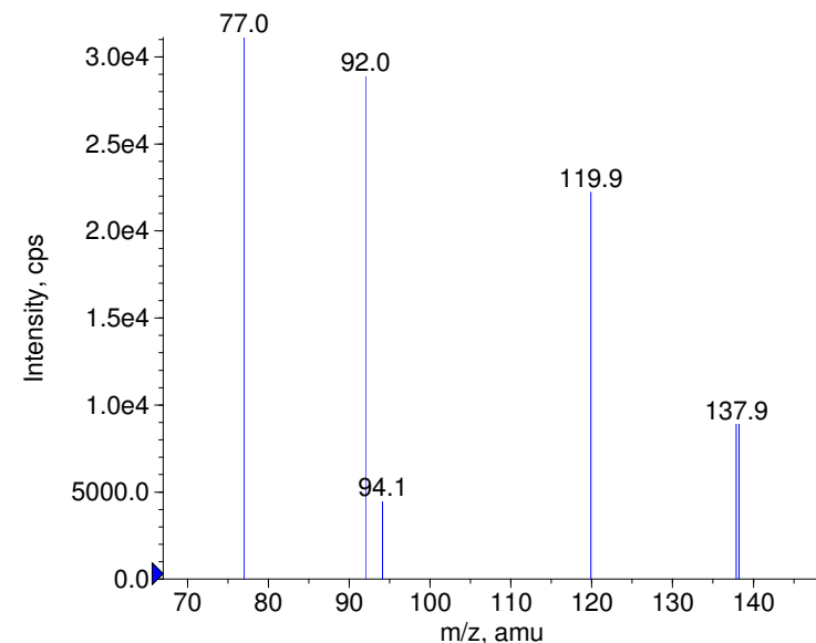
+ Propham Prec(180.0) CE(99.0) RT(0.6)
