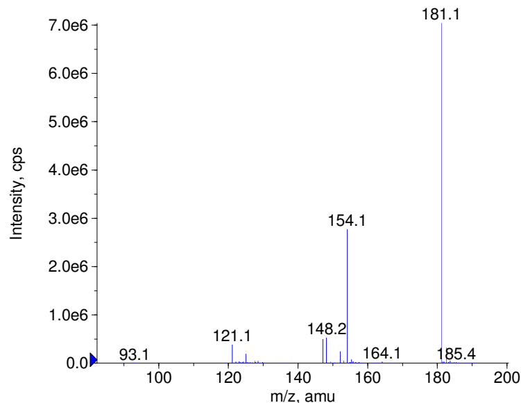
+ Protionamide Prec(181.0) CE(50.0) RT(1.0)
