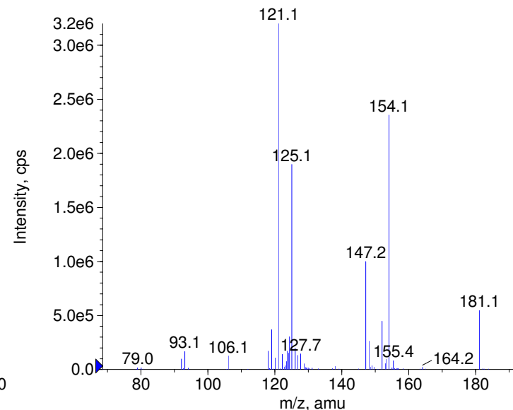
+ Protionamide Prec(181.0) CE(99.0) RT(1.1)
