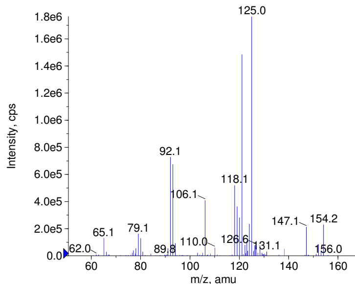
+ Protionamide Prec(181.0) CE(50.0) RT(1.0)
