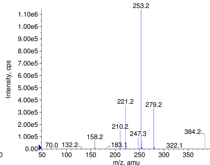
+ Quetiapine Prec(384.0) CE(99.0) RT(0.8)
