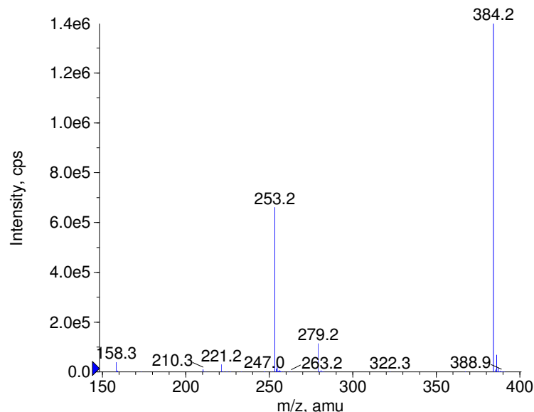
+ Quetiapine Prec(384.0) CE(50.0) RT(0.8)
