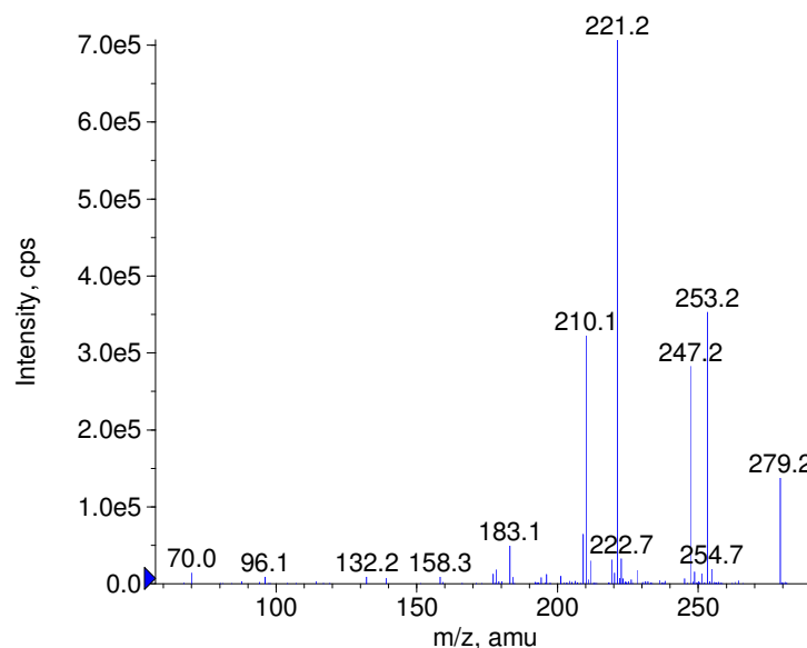
+ Quetiapine Prec(384.0) CE(50.0) RT(0.8)
