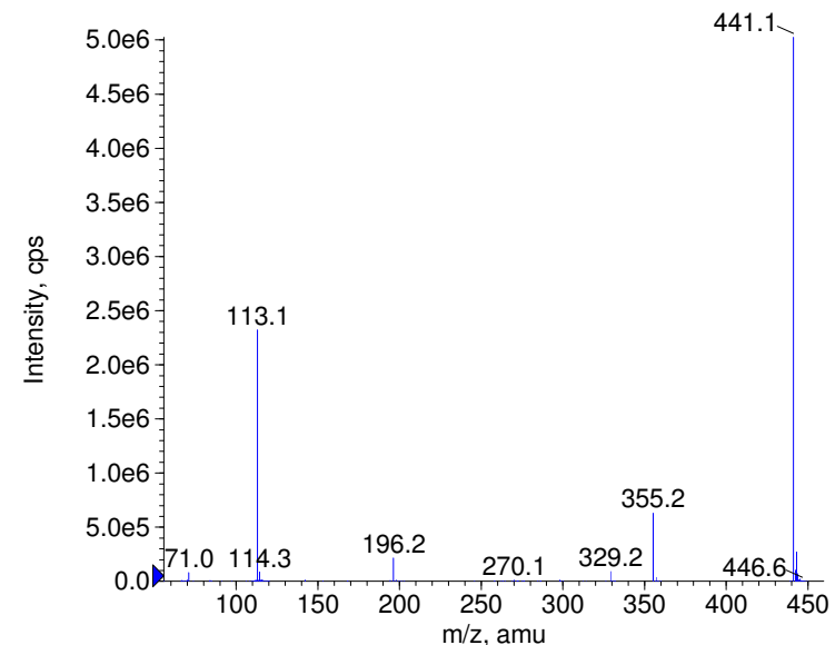
+ Sertindole Prec(441.0) CE(99.0) RT(0.8)
