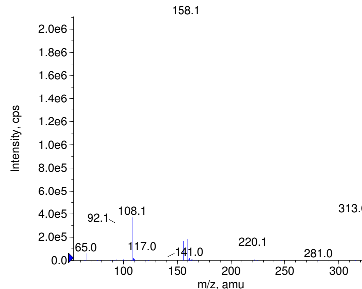
■ + Sulfacloamide Prec(313.0) CE(99.0) RT(0.8)
