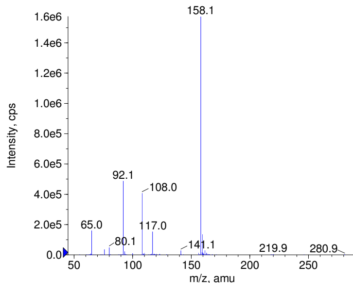
■ + Sulfacloamide Prec(313.0) CE(50.0) RT(0.8)
