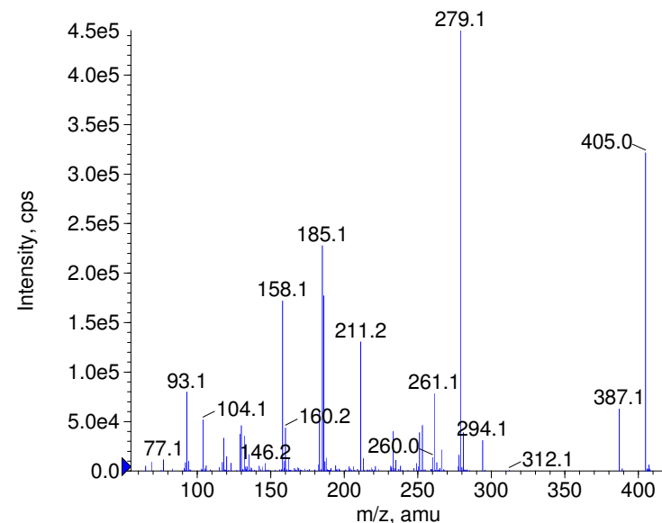
■ + Sulfinpyrazone Prec(405.0) CE(99.0) RT(0.9)
