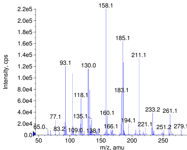
■ + Sulfinpyrazone Prec(405.0) CE(50.0) RT(0.9)
