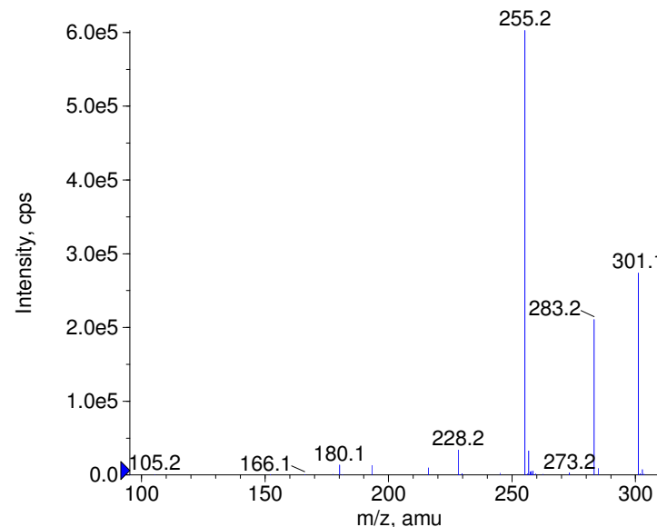
+ Temazepam Prec(301.0) CE(50.0) RT(1.0)
