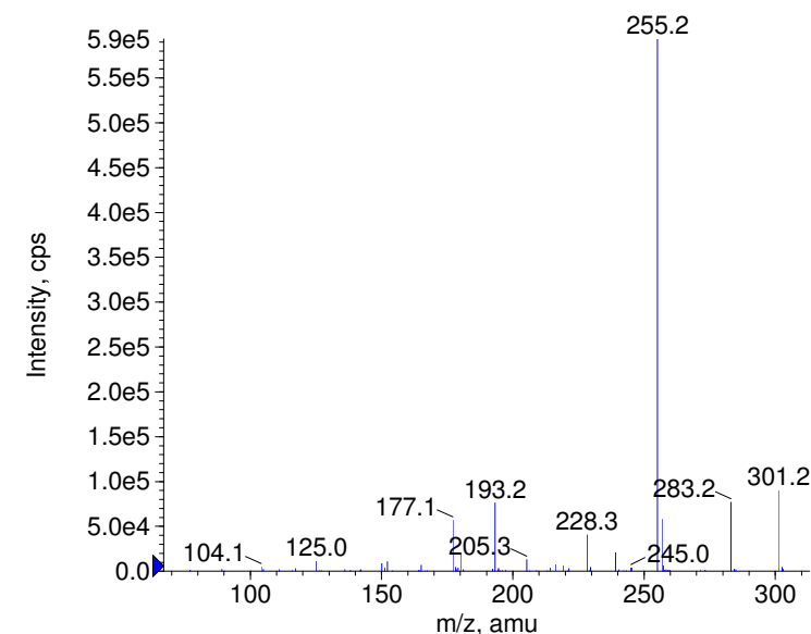
+ Temazepam Prec(301.0) CE(99.0) RT(1.0)
