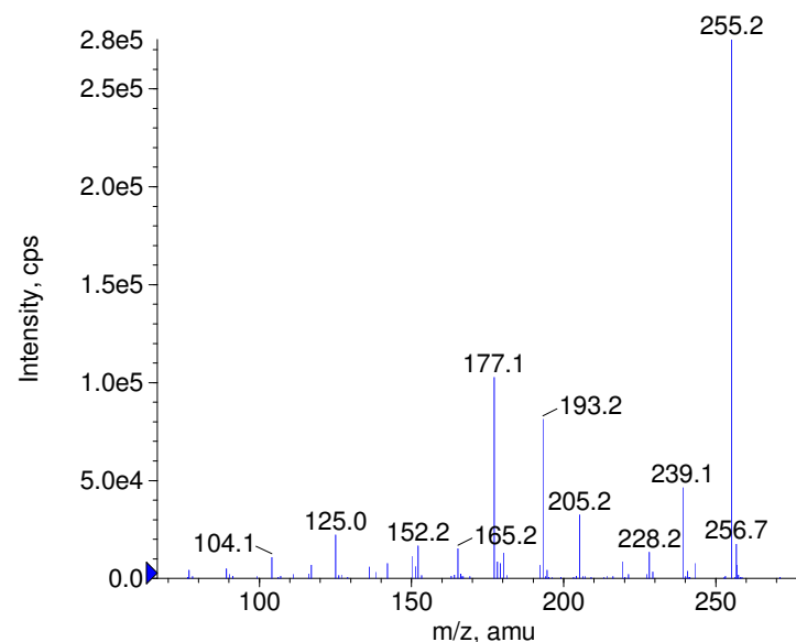
+ Temazepam Prec(301.0) CE(50.0) RT(1.0)
