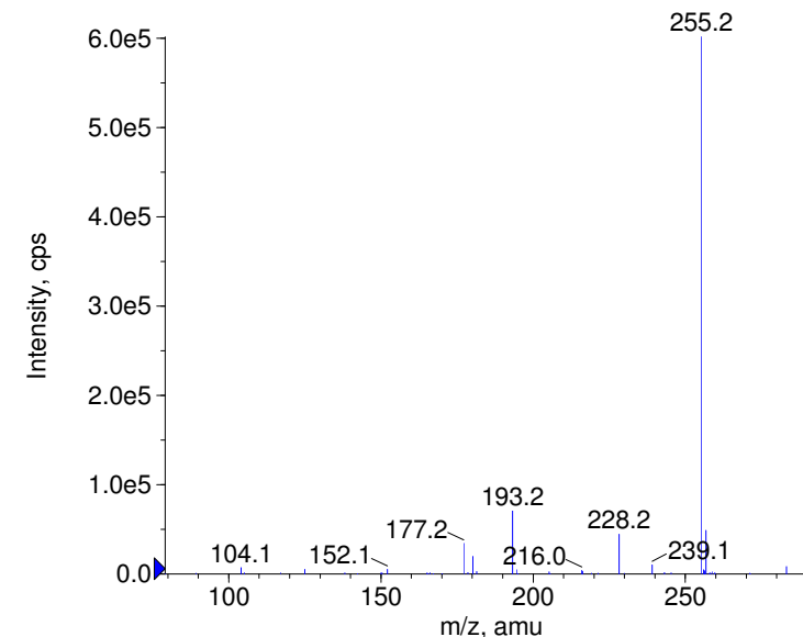
+ Temazepam Prec(301.0) CE(99.0) RT(1.0)
