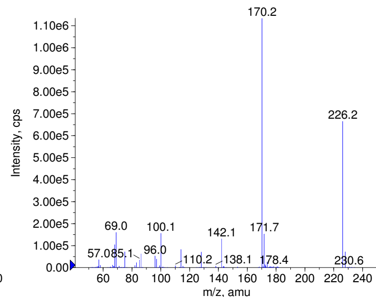
+ Terbumeton Prec(226.0) CE(99.0) RT(1.1)
