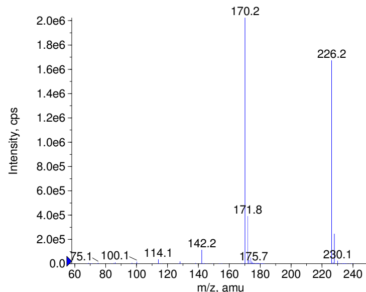
+ Terbumeton Prec(226.0) CE(50.0) RT(1.1)
