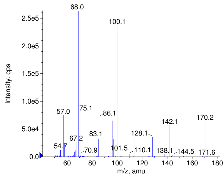
+ Terbumeton Prec(226.0) CE(50.0) RT(1.1)
