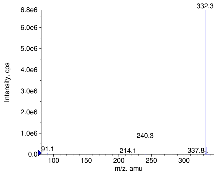
+ Tetramethrin Prec(332.0) CE(50.0) RT(0.9)
