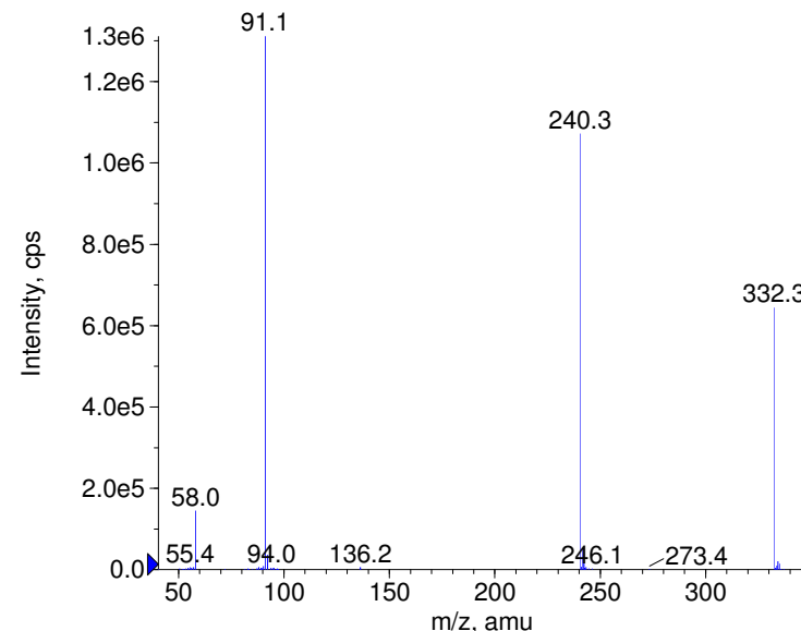
+ Tetramethrin Prec(332.0) CE(99.0) RT(0.9)
