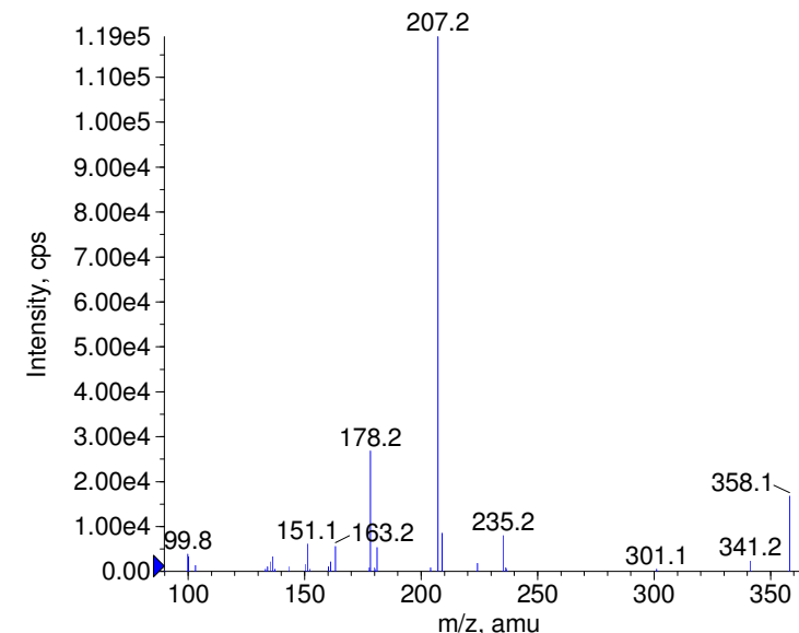
+ Theodrenaline Prec(376.0) CE(99.0) RT(0.7)
