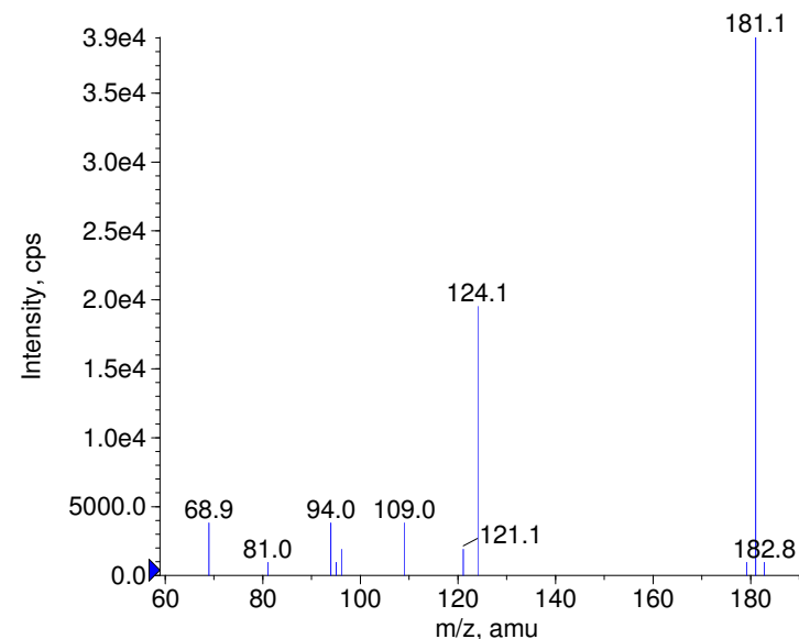
■ + Theophylline Prec(181.0) CE(99.0) RT(0.7)
