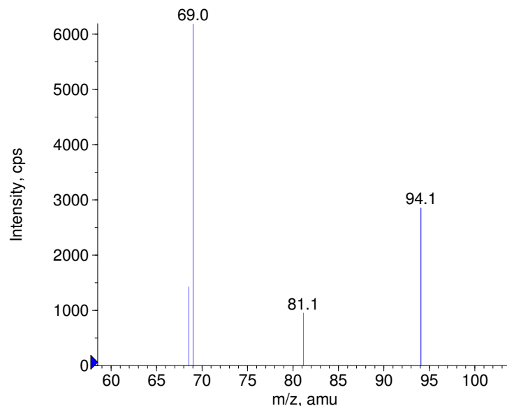
■ + Theophylline Prec(181.0) CE(50.0) RT(0.7)
