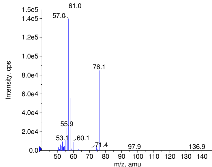
+ Thiofanox Prec(219.0) CE(99.0) RT(0.8)
