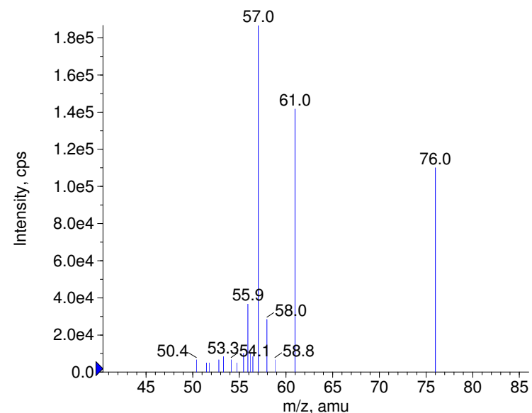
+ Thiofanox Prec(219.0) CE(99.0) RT(0.8)
