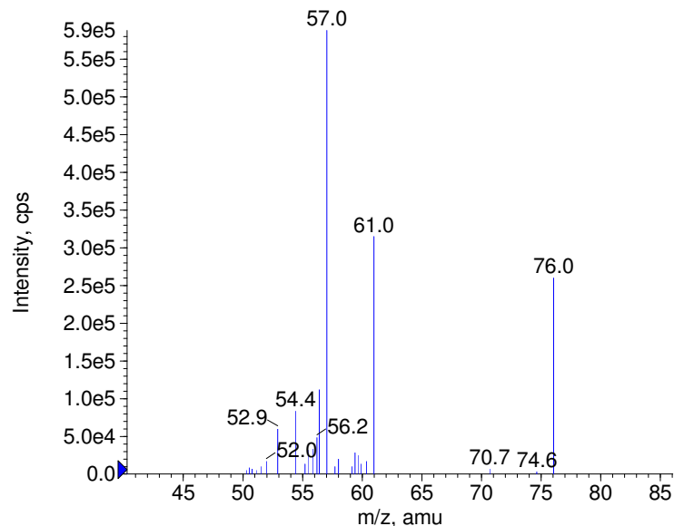
+ Thiofanox Prec(219.0) CE(50.0) RT(0.8)
