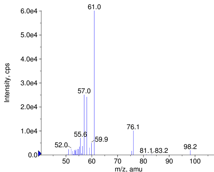
+ Thiofanox Prec(219.0) CE(50.0) RT(0.8)
