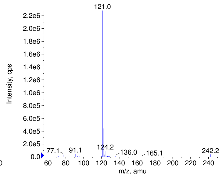
+ Thonzylamine Prec(287.0) CE(99.0) RT(0.9)
