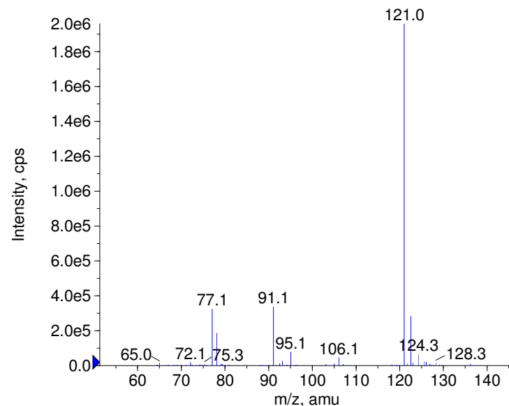
+ Thonzylamine Prec(287.0) CE(50.0) RT(0.9)
