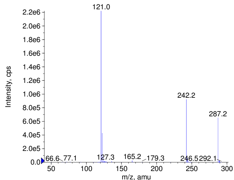
+ Thonzylamine Prec(287.0) CE(50.0) RT(0.9)
