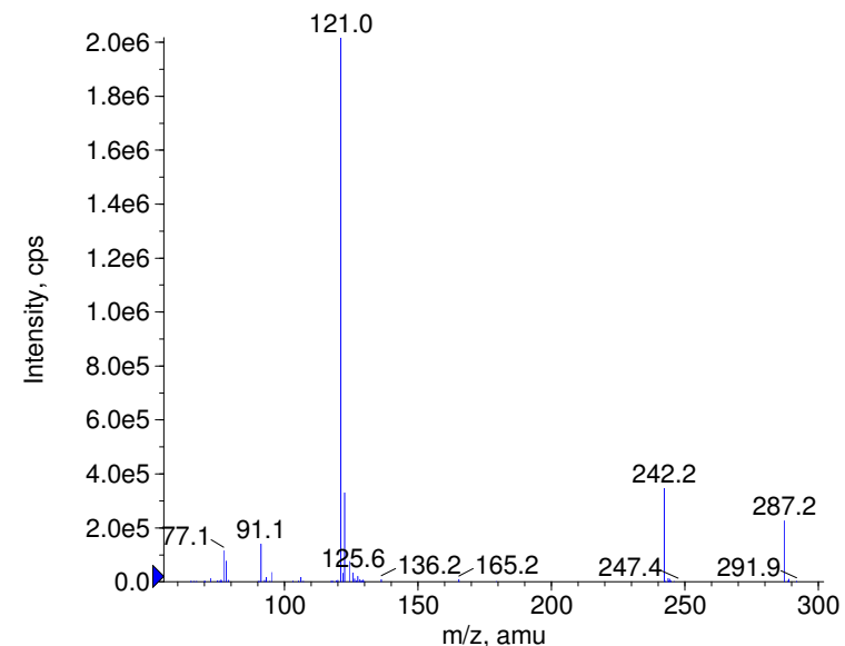
+ Thonzylamine Prec(287.0) CE(99.0) RT(0.9)
