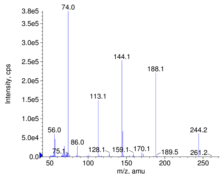
+ Timolol Prec(317.0) CE(50.0) RT(0.7)
