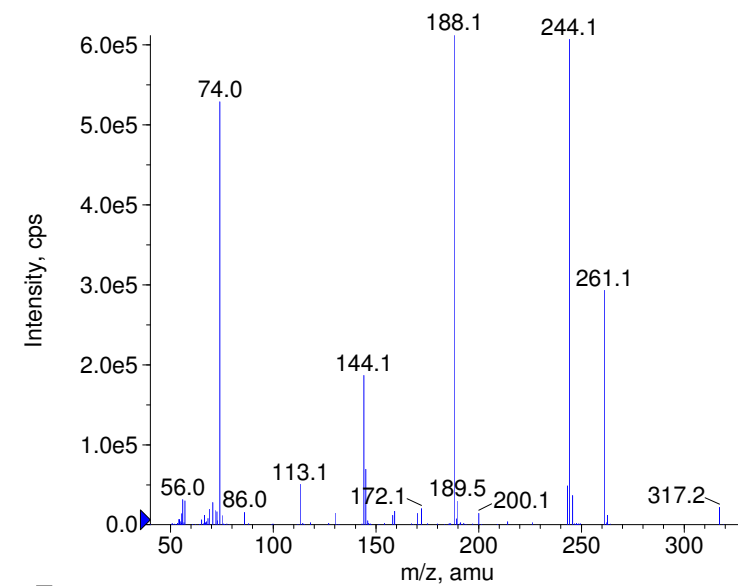
+ Timolol Prec(317.0) CE(99.0) RT(0.8)
