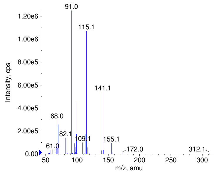
■ + Tolazamide Prec(312.0) CE(35.0) RT(0.9)
