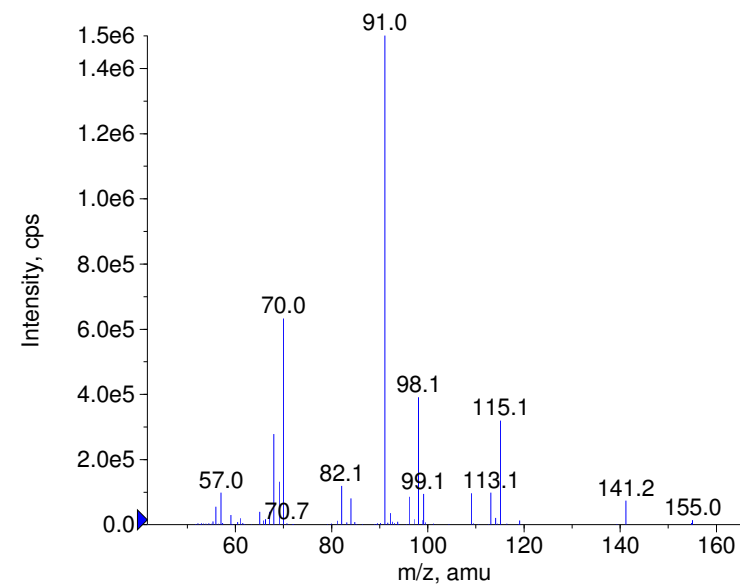
■ + Tolazamide Prec(312.0) CE(50.0) RT(0.9)
