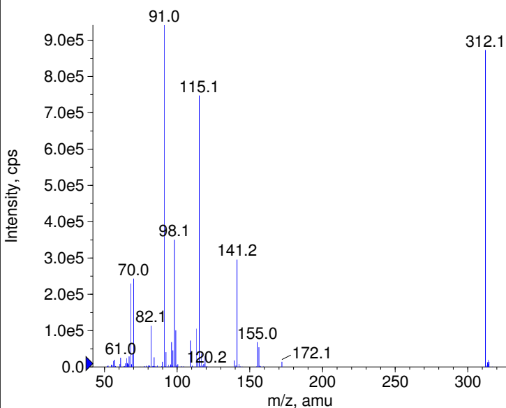
■ + Tolazamide Prec(312.0) CE(99.0) RT(1.0)
