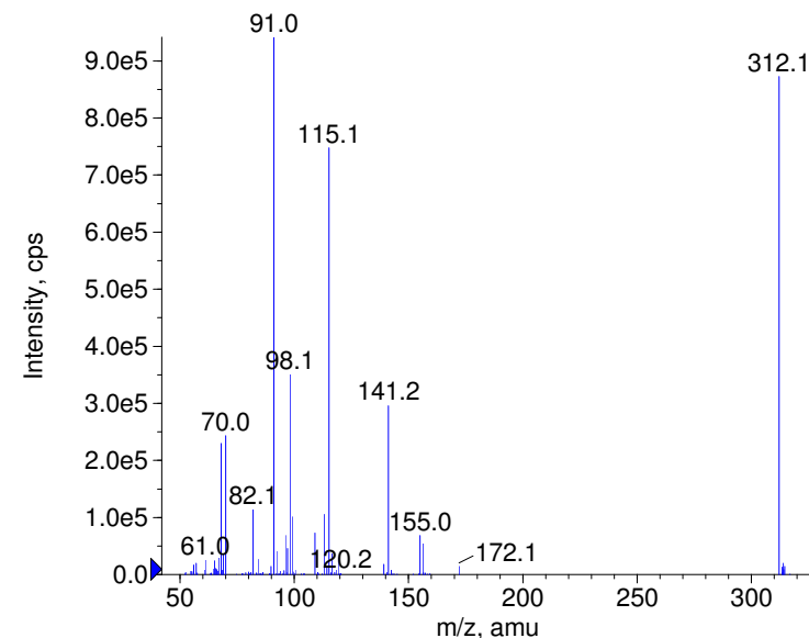
+ Tolazamide Prec(312.0) CE(99.0) RT(1.0)
