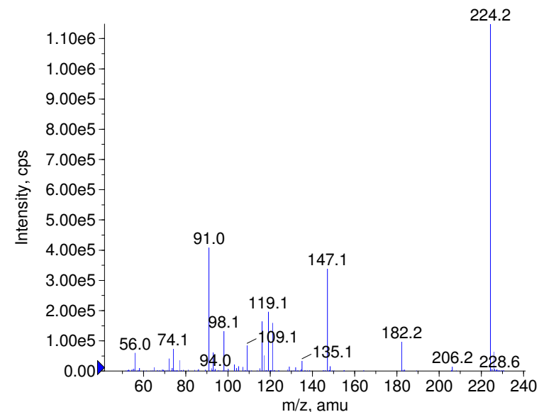
+ Toliprolol Prec(224.0) CE(99.0) RT(0.7)
