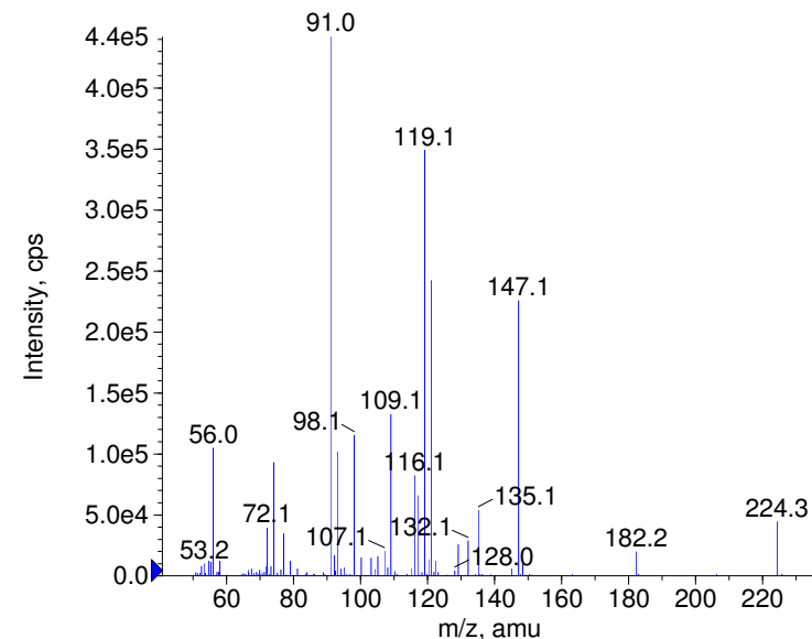
+ Toliprolol Prec(224.0) CE(99.0) RT(0.7)
