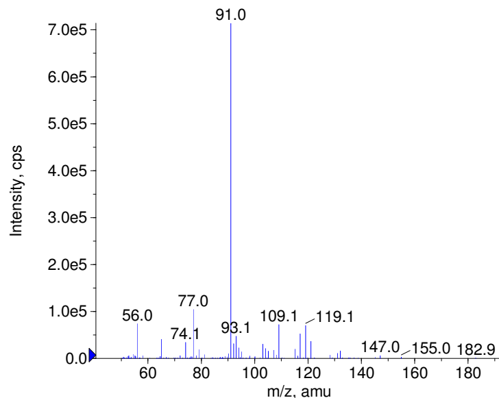
+ Toliprolol Prec(224.0) CE(50.0) RT(0.7)
