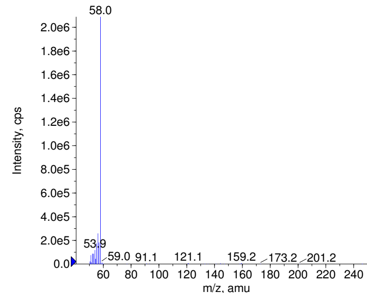
+ Tramadol Prec(264.0) CE(99.0) RT(0.7)
