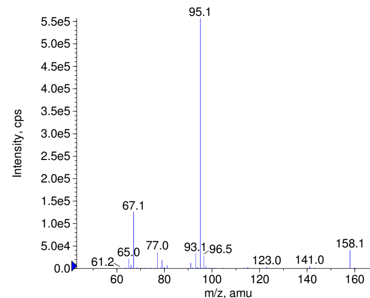
+ Tranexamic acid Prec(158.0) CE(99.0) RT(0.8)
