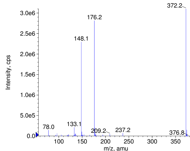
+ Trazodone Prec(372.0) CE(99.0) RT(0.7)
