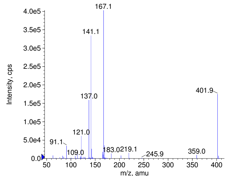
+ Triasulfuron Prec(402.0) CE(99.0) RT(0.9)
