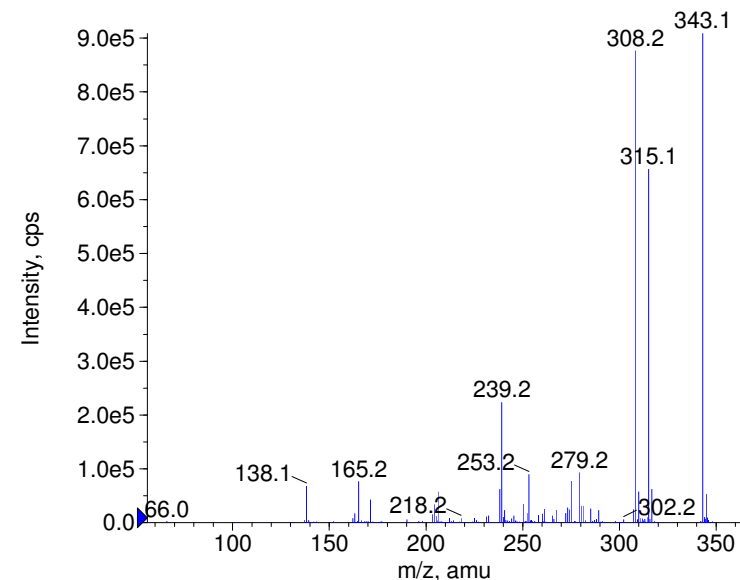
+ Triazolam Prec(343.0) CE(99.0) RT(1.0)
