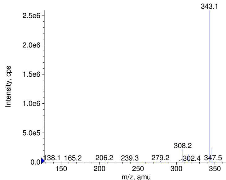
+ Triazolam Prec(343.0) CE(50.0) RT(1.0)
