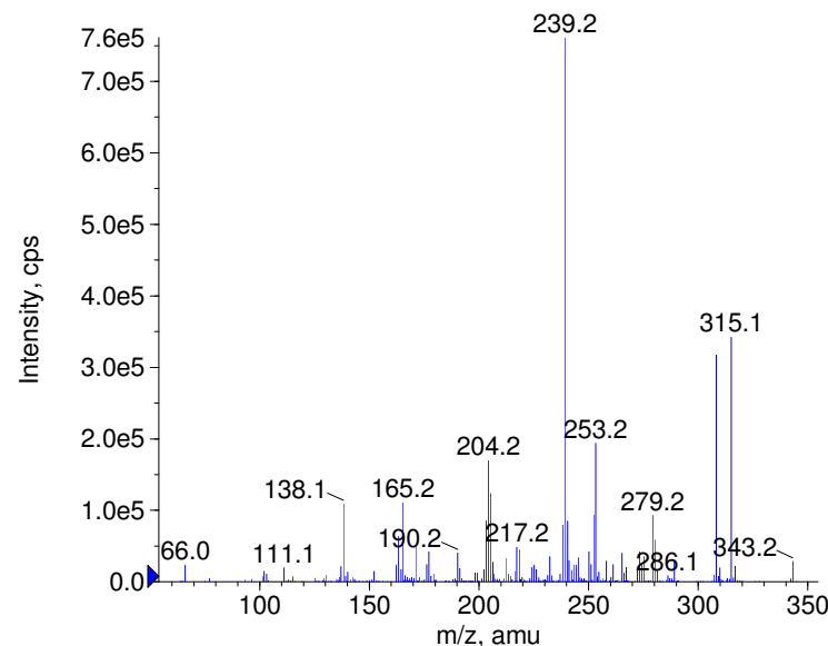
+ Triazolam Prec(343.0) CE(50.0) RT(1.0)
