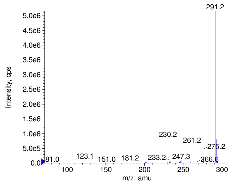
+ Trimethoprim Prec(291.0) CE(50.0) RT(0.7)
