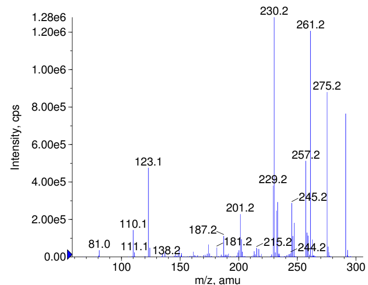
+ Trimethoprim Prec(291.0) CE(99.0) RT(0.7)
