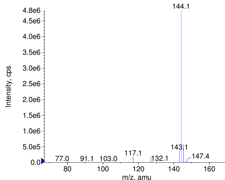
+ Tryptamine Prec(161.0) CE(50.0) RT(0.8)
