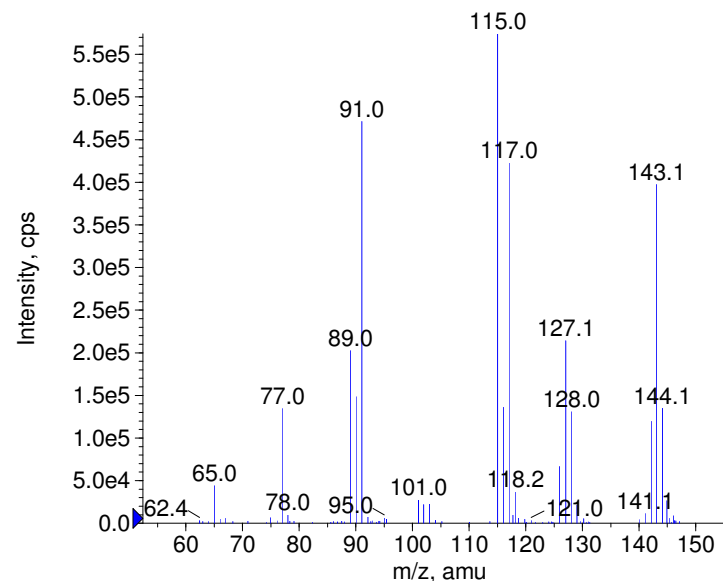
+ Tryptamine Prec(161.0) CE(50.0) RT(0.8)
