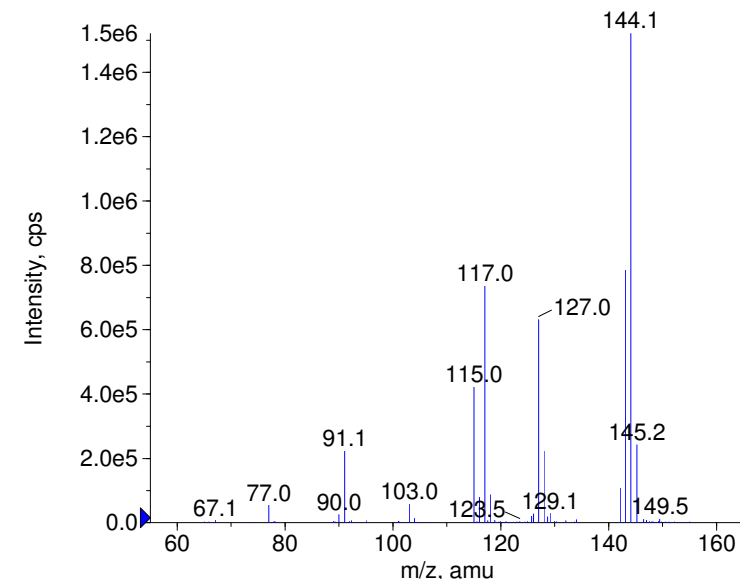
+ Tryptamine Prec(161.0) CE(99.0) RT(0.8)
