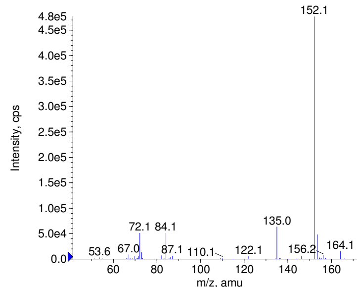
+ Valacyclovir Prec(325.0) CE(99.0) RT(0.9)
