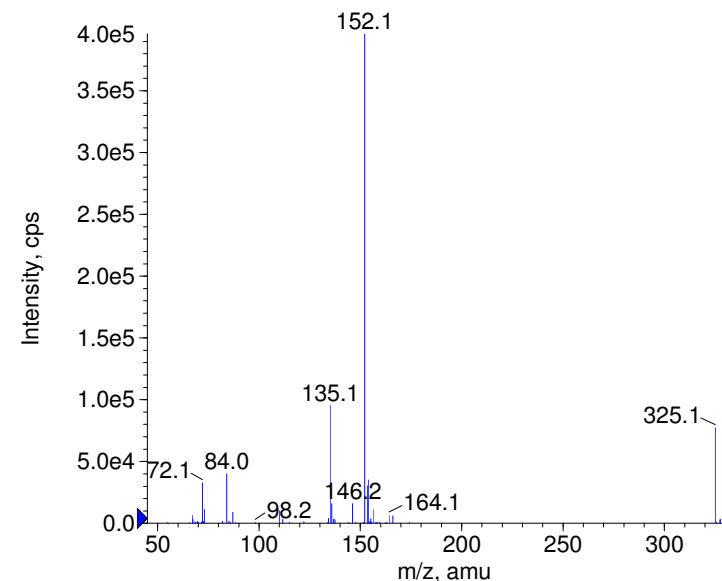
+ Valacyclovir Prec(325.0) CE(99.0) RT(0.9)
