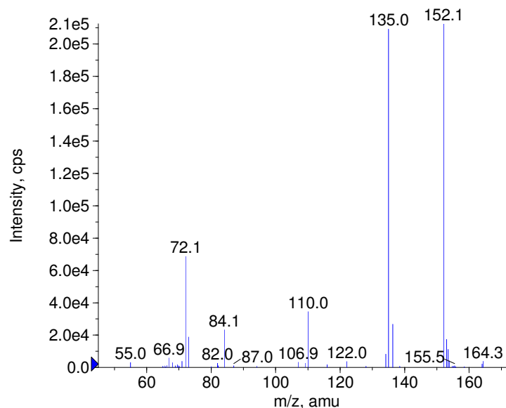
+ Valacyclovir Prec(325.0) CE(50.0) RT(0.8)
