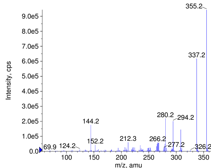
+ Vincamine Prec(355.0) CE(99.0) RT(0.8)
